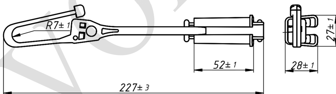
Рисунок 1. Зажим анкерный VS-P-25-90
