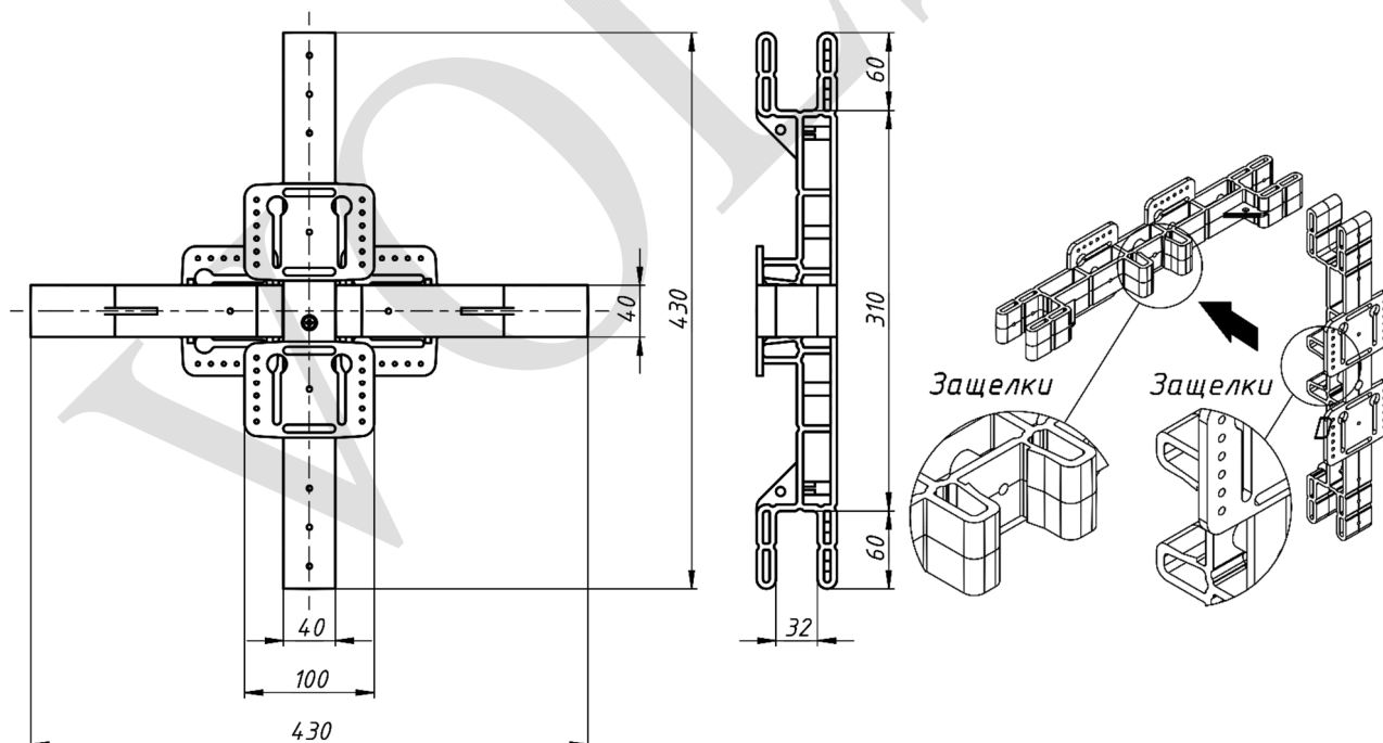
Рисунок 1. VS-УПМК-300П
